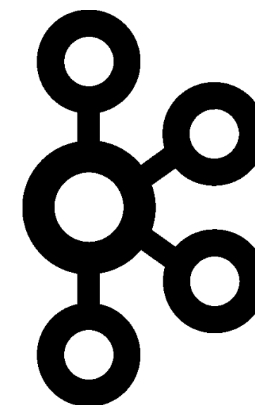
Apache Kafka
